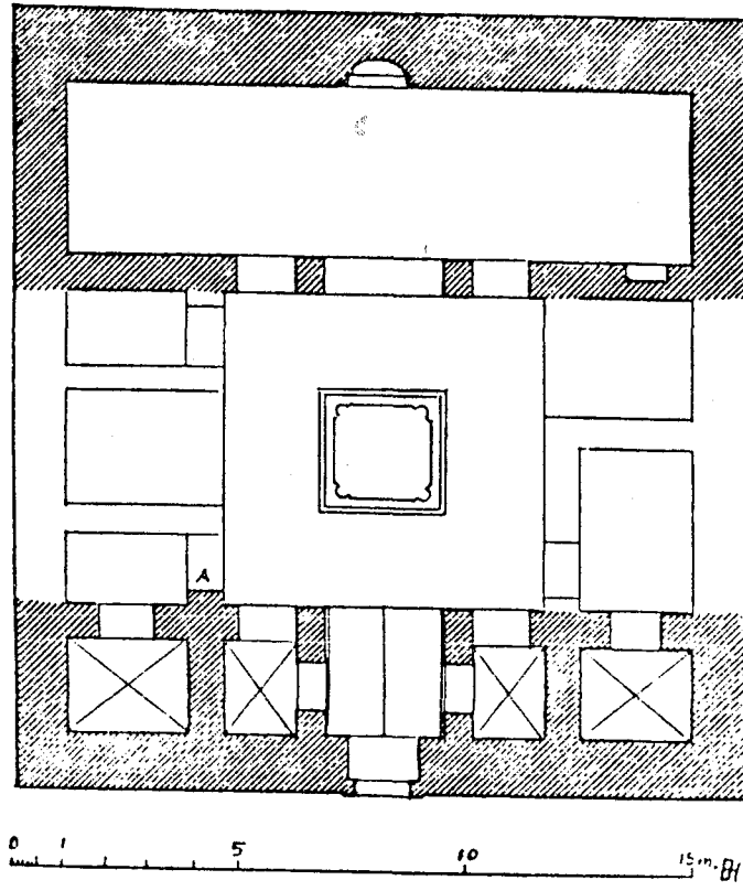
Plân 1. Daru'l-hadis en-Nuriyye'nin plânı.
