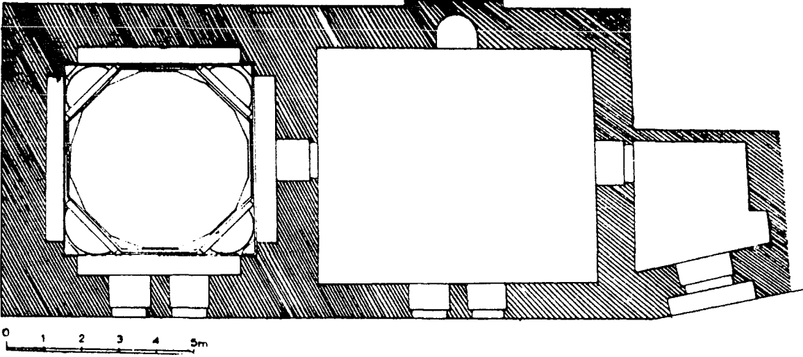
Plân 2. Daru'l-hadis el-Eşrefiyye el-Berrâniyye'nin plânı.
